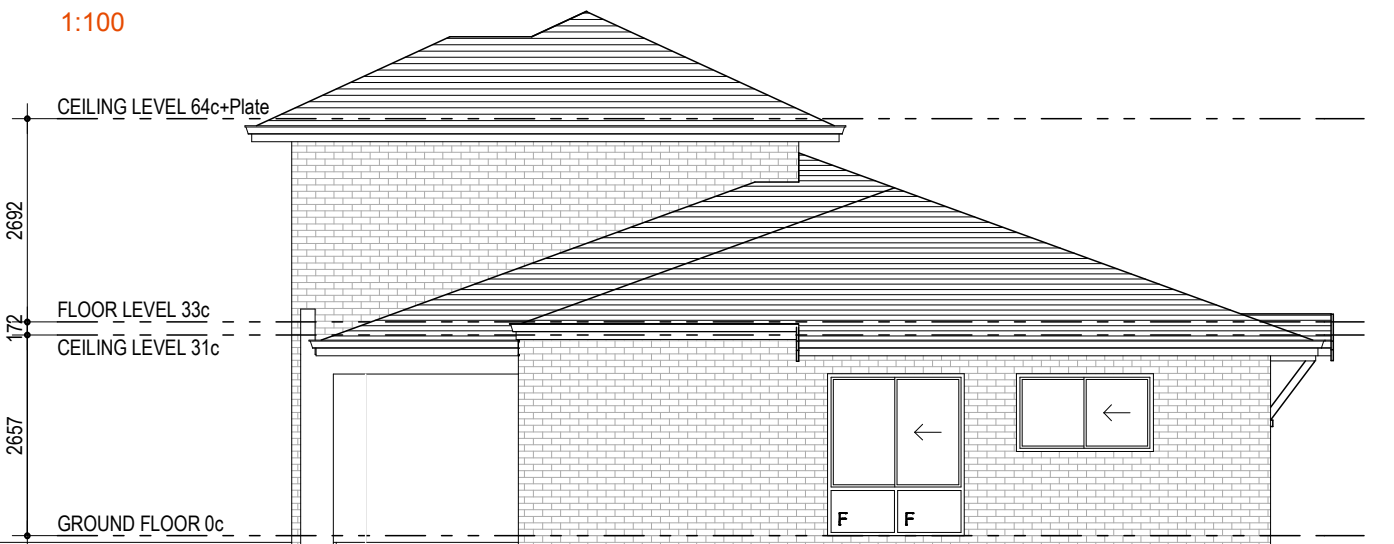
ELEVATION 4
