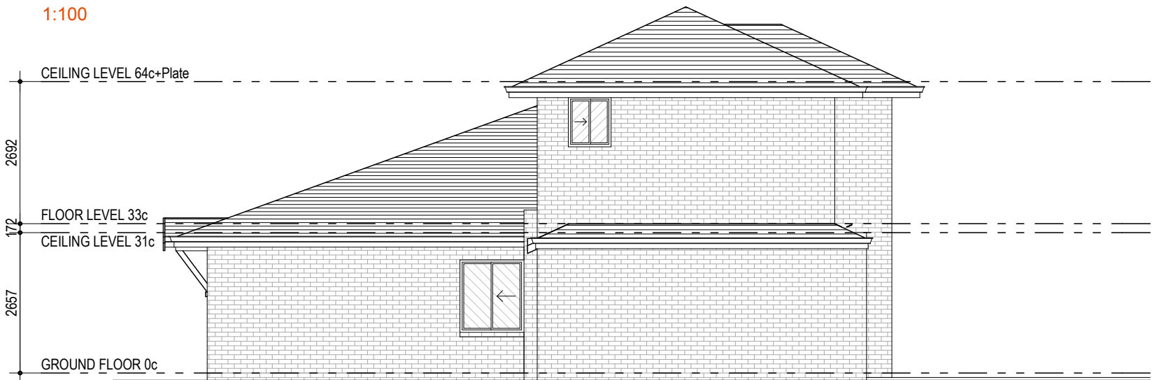
ELEVATION 2
