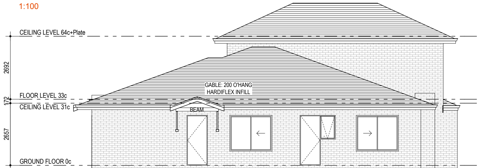
ELEVATION 3
