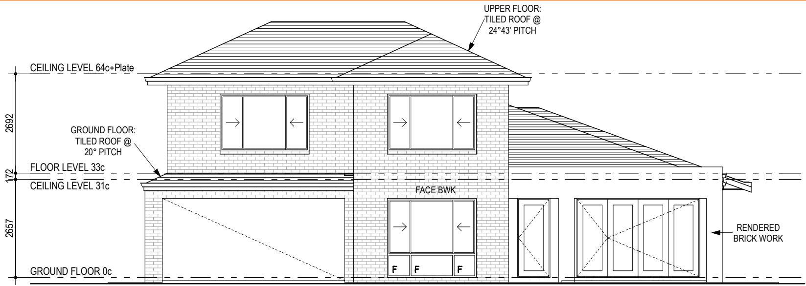
ELEVATION 1
