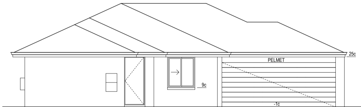
ELEVATION 2
