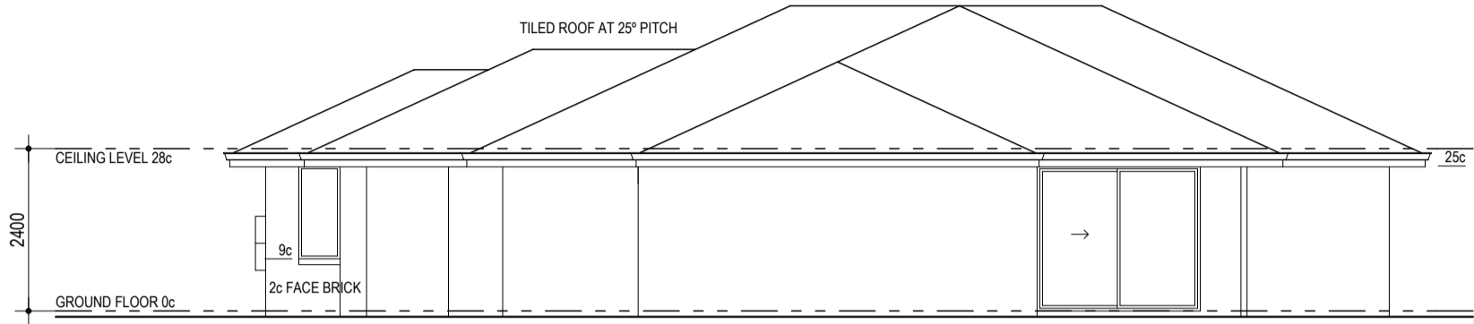
ELEVATION 1
