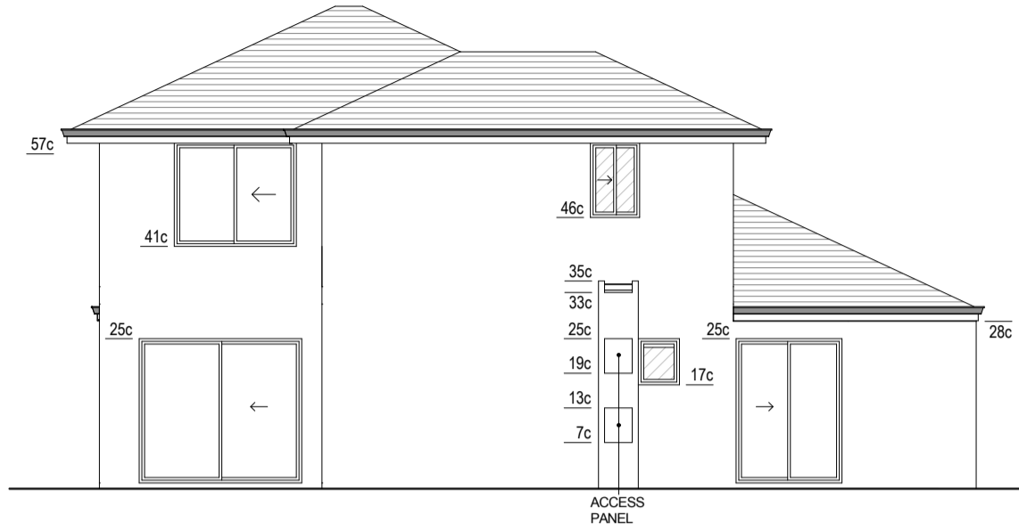
ELEVATION A
