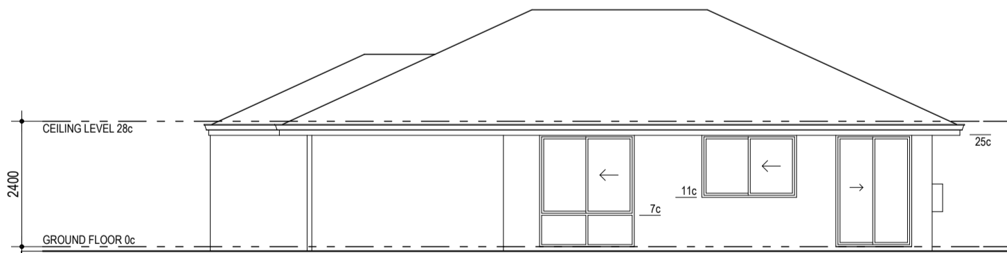
ELEVATION 4
