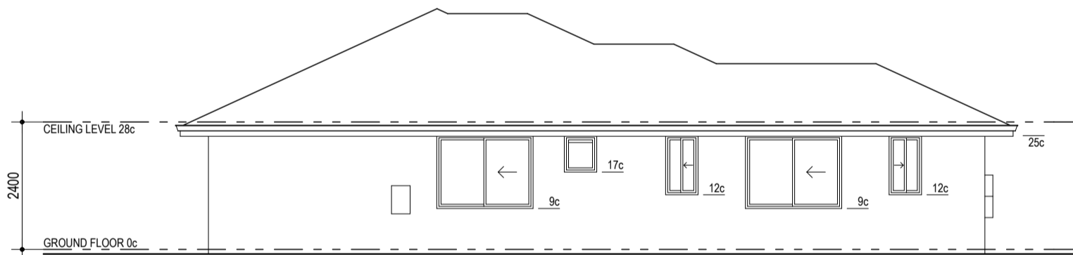
ELEVATION 3
