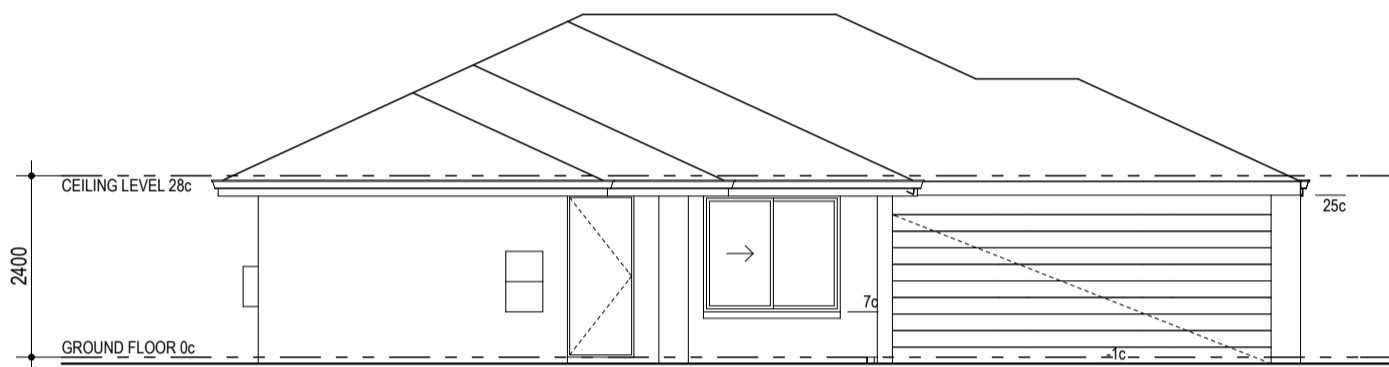
ELEVATION 2
