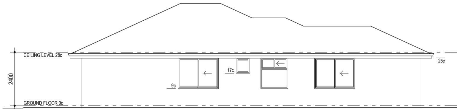
ELEVATION 3
