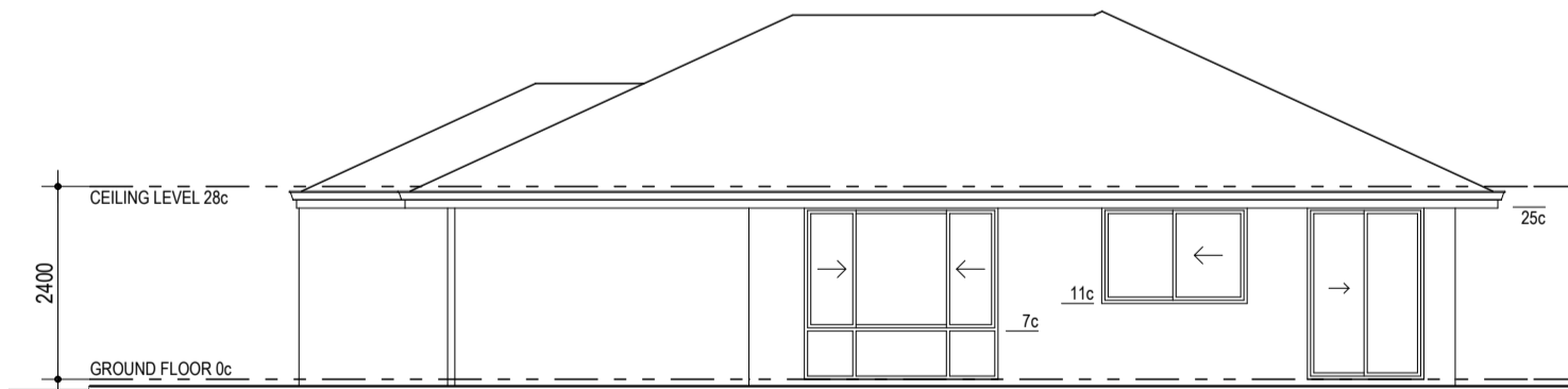
ELEVATION 4
