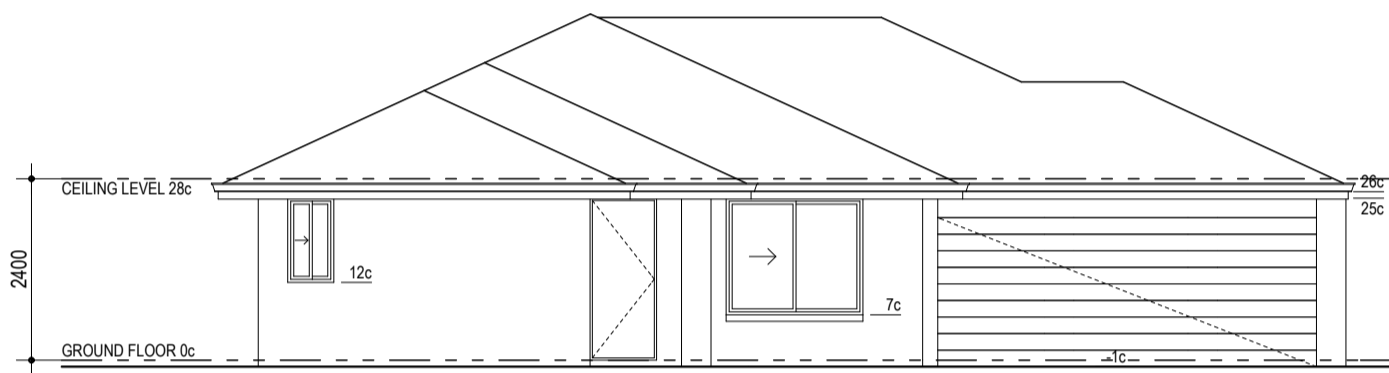
ELEVATION 2
