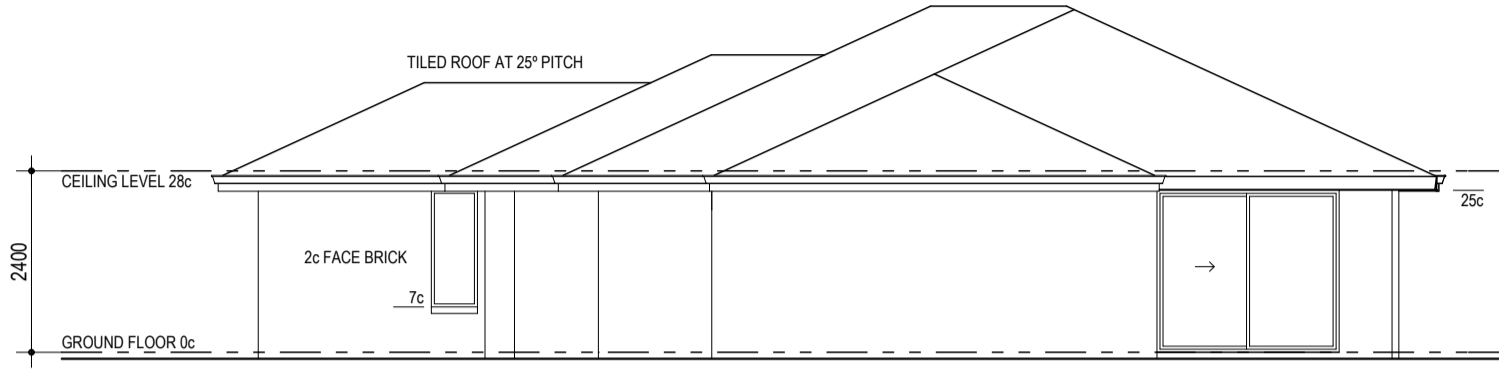
ELEVATION 1
