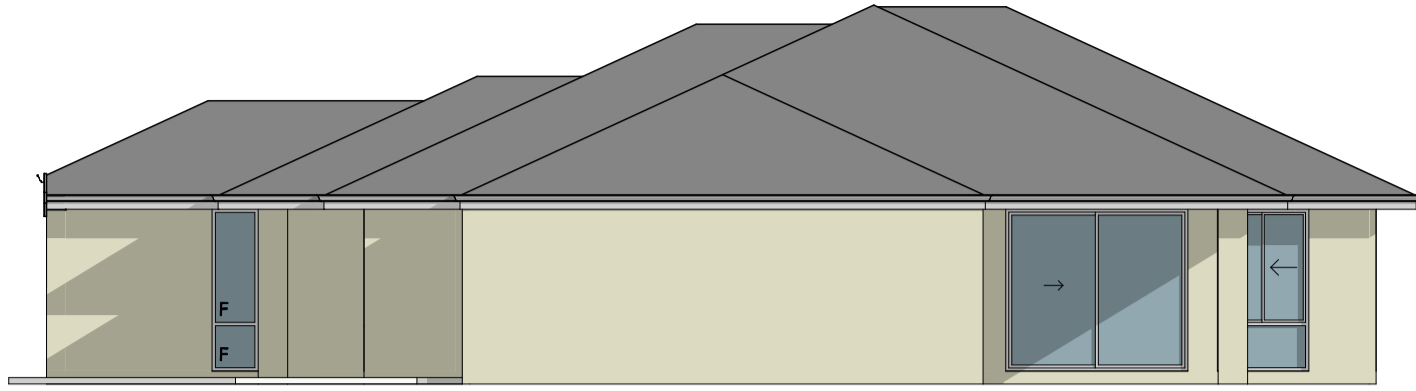
ELEVATION A
